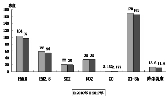
图三 2017 年我市主要污染物浓度同比图
