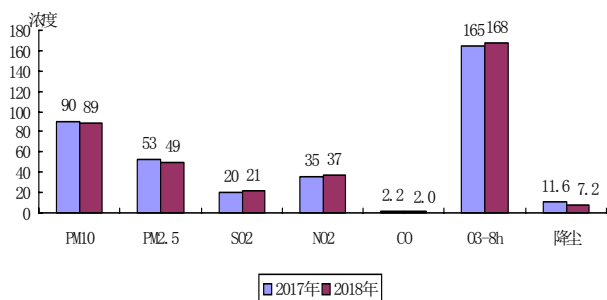
图三 2018年我市主要污染物浓度同比图
