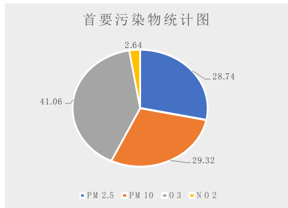
图二 2018年各类首要污染物所占比例图
