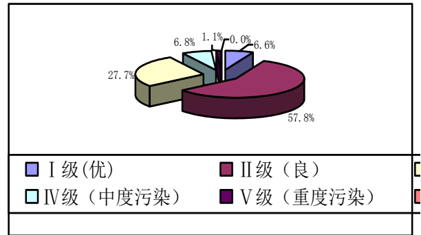
图一 2018年各类级别天数所占比例图
