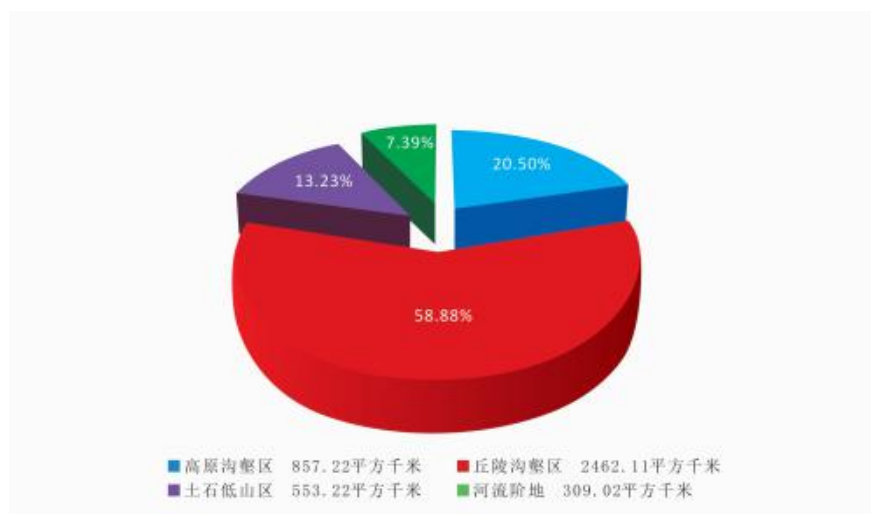
富县 2010 年地貌类型示意图
