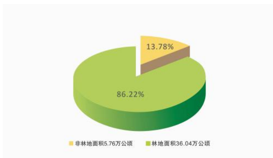
富县 2006 年森林资源调整结果示意图
