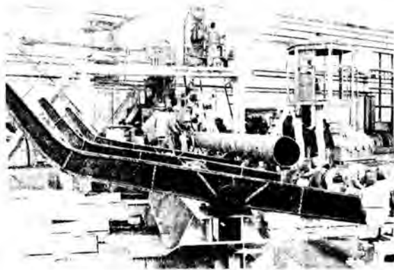
宝鸡石油钢管厂双面埋弧焊管二号机组
