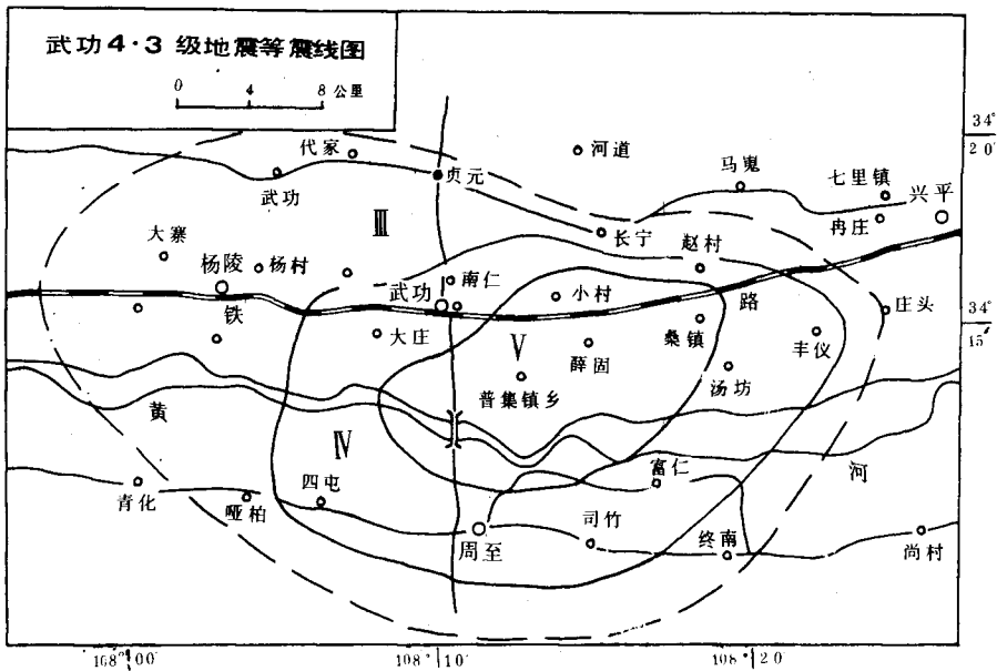
图 武功地震等烈度线图
